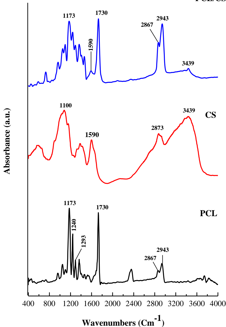
شکل ۵- طیف مادون قرمز پلی کاپرولاکتون، کیتوسان و پلی کاپرولاکتون: کیتوسان
