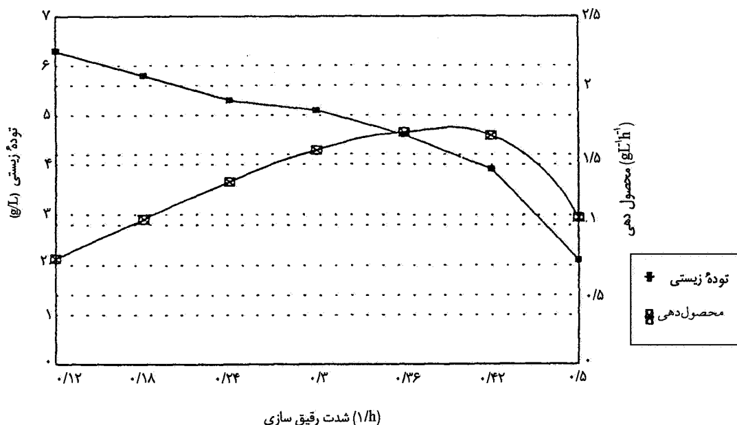
شکل ۷- تغییرات توده زیستی و محصول دهی با شدت رقیق سازی. دمای 34^{\circ}\text{C} ، شدت هوادهی ۲۷.۷.م، دور هم‌زن ۸۰۰ r.p.m pH اولیه محیط کشت ۳/۵
