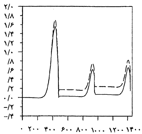
ب - توزیع کرنش طولی مسافت طی شده توسط نوار [ mm ]
