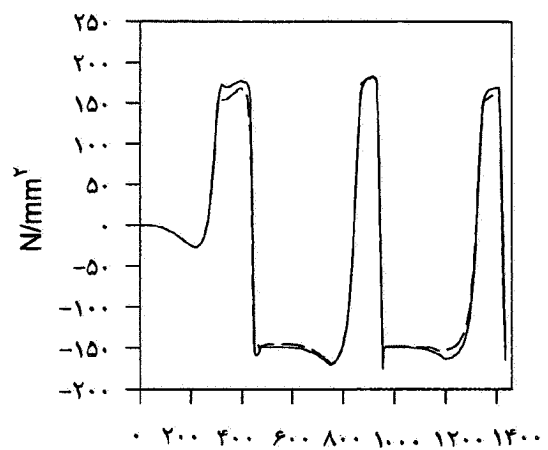
الف - توزیع تنش طولی مسافت طی شده توسط نوار [ mm ]
