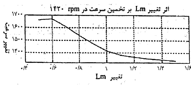
شکل ۸- اثر تغییر L_m بر روی تخمینگر سرعت در 1420 rpm
