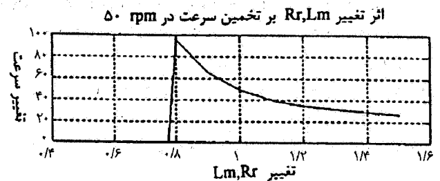
شکل ۱۳- اثر تغییر Lm, Rr بر روی تخمینگر سرعت در 50 \text{ rpm}
