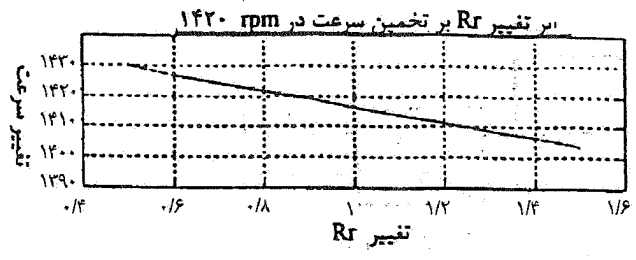
شکل ۷- اثر تغییر R_r بر روی تخمینگر سرعت در 1420 rpm
