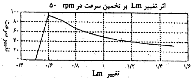
شکل ۱۱- اثر تغییر Lm بر روی تخمینگر سرعت در 50 \text{ rpm}
