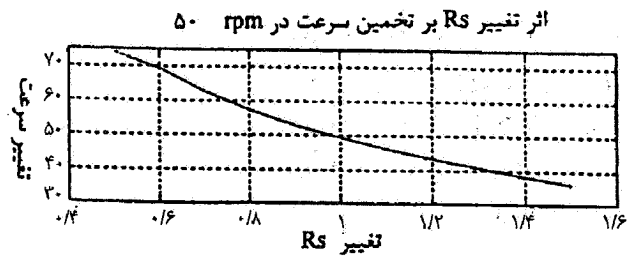
شکل ۹- اثر تغییر Rs بر روی تخمینگر سرعت در 50 \text{ rpm}
