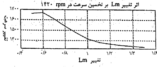
شکل ۸- اثر تغییر Lm بر روی تخمینگر سرعت در 1420 rpm
