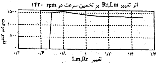
شکل ۱۲- اثر تغییر Lm, Rr بر روی تخمینگر سرعت در 1420 \text{ rpm}
