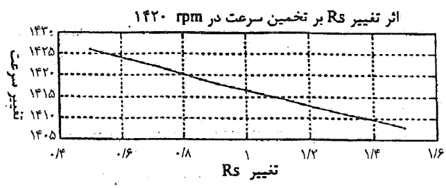
شکل ۶- اثر تغییر R_s بر روی تخمینگر سرعت در 1420 rpm
