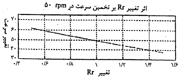
شکل ۱۰- اثر تغییر Rr بر روی تخمینگر سرعت در 50 \text{ rpm}
