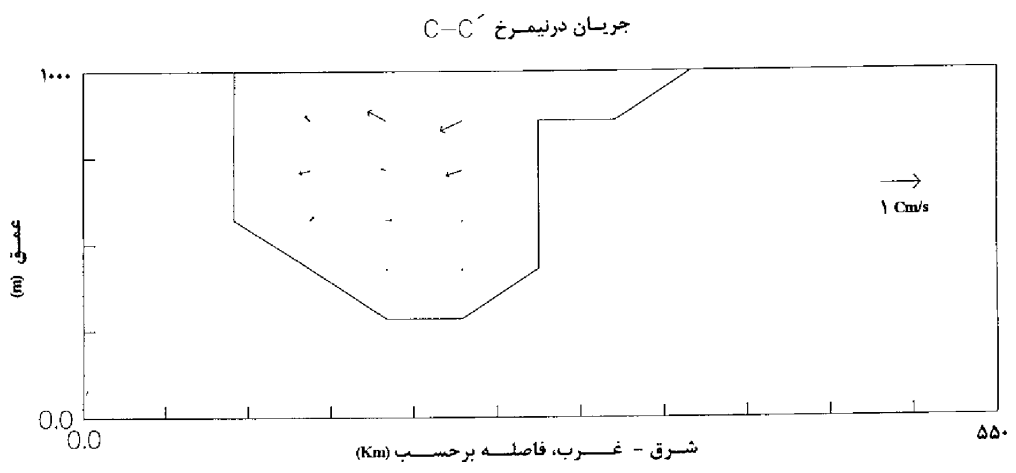
شکل ۶- جریانهای اصلی در دریای خزر حاصل از مدل عددی در حالت پایا در برش عرضی C-C'
