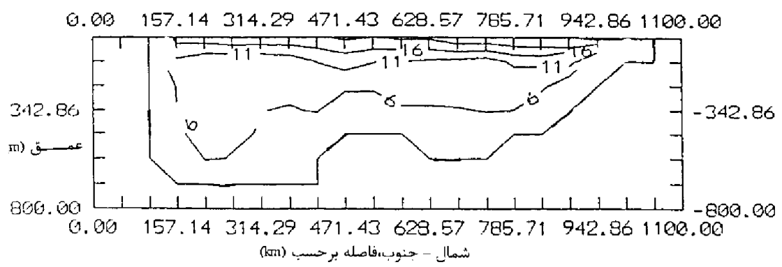
شکل ۱۱-الف- نیمرخ دما در برش N-S حاصل از مشاهدات نیمرخ دما (N-S)
