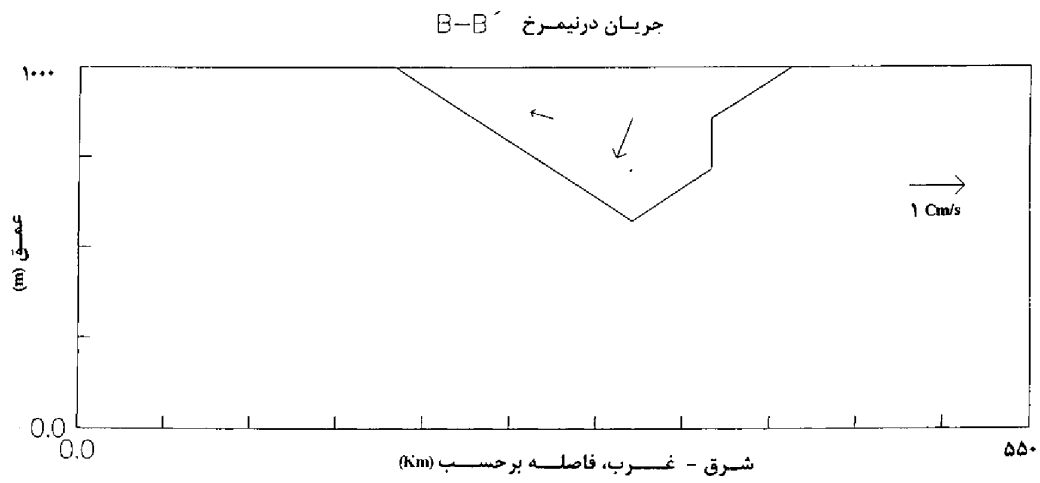
شکل ۵- جریانهای اصلی در دریای خزر حاصل از مدل عددی در حالت پایا در برش عرضی B-B'
