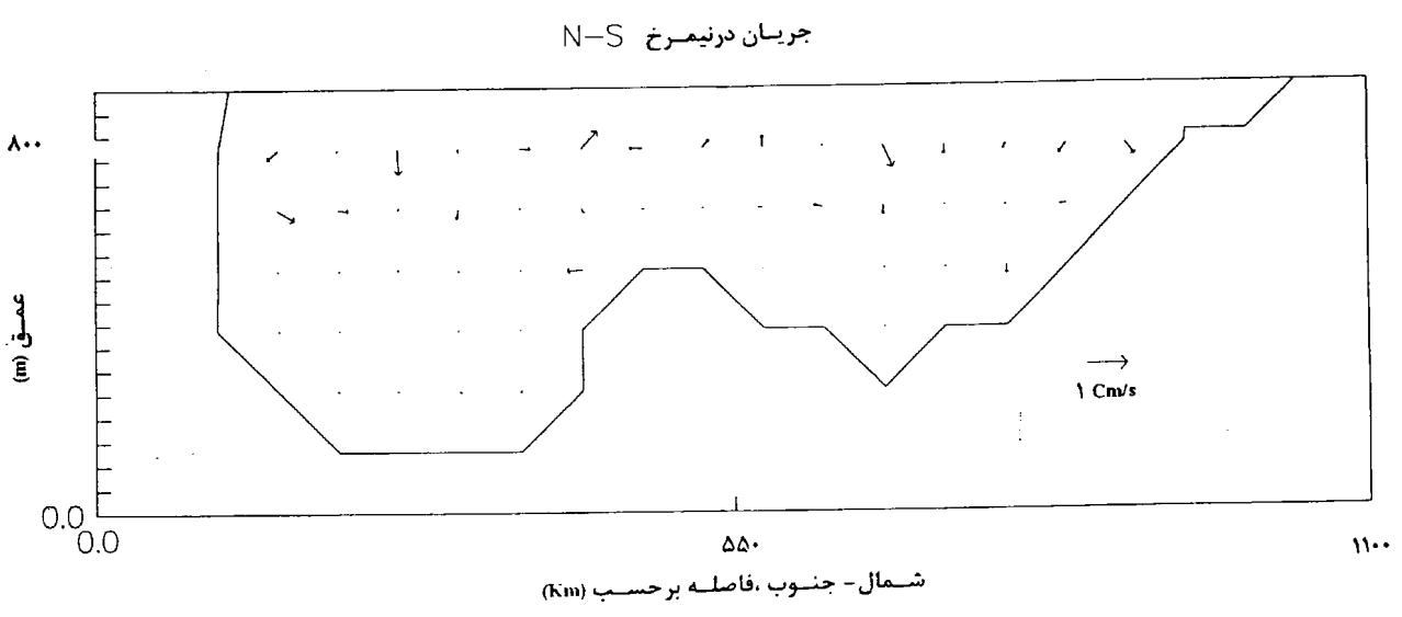
شکل ۷- جریانهای اصلی در دریای خزر حاصل از مدل عددی در حالت پایا در برش طولی N-S
