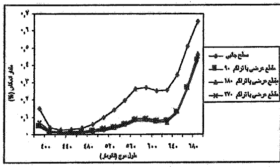
شکل ۶- منحنی انعکاس طیفی نمونه شماره ۲ در امتداد طولی و مقطع عرضی با تراکمهای مختلف
