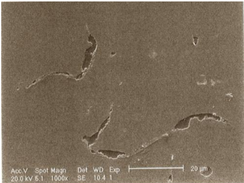
شکل ۵ - تصویر میکروسکوپی SEM از لایه پوششی SiO 2 بر روی زیرلایه شیشه‌ای، آلودگیهای سطحی بر روی زیرلایه باعث عدم تشکیل پوشش در بعضی از قسمتهای آن شده است.
