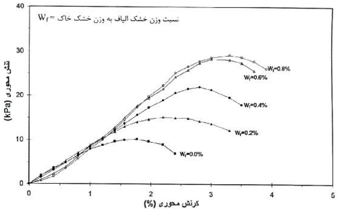
شکل ۱۱- تغییرات تنش بر حسب کرنش محوری در آزمایش تک محوری برای درصدهای وزنی عناصر تسلیح W_f و نسبت اضلاع عناصر A_R=1
