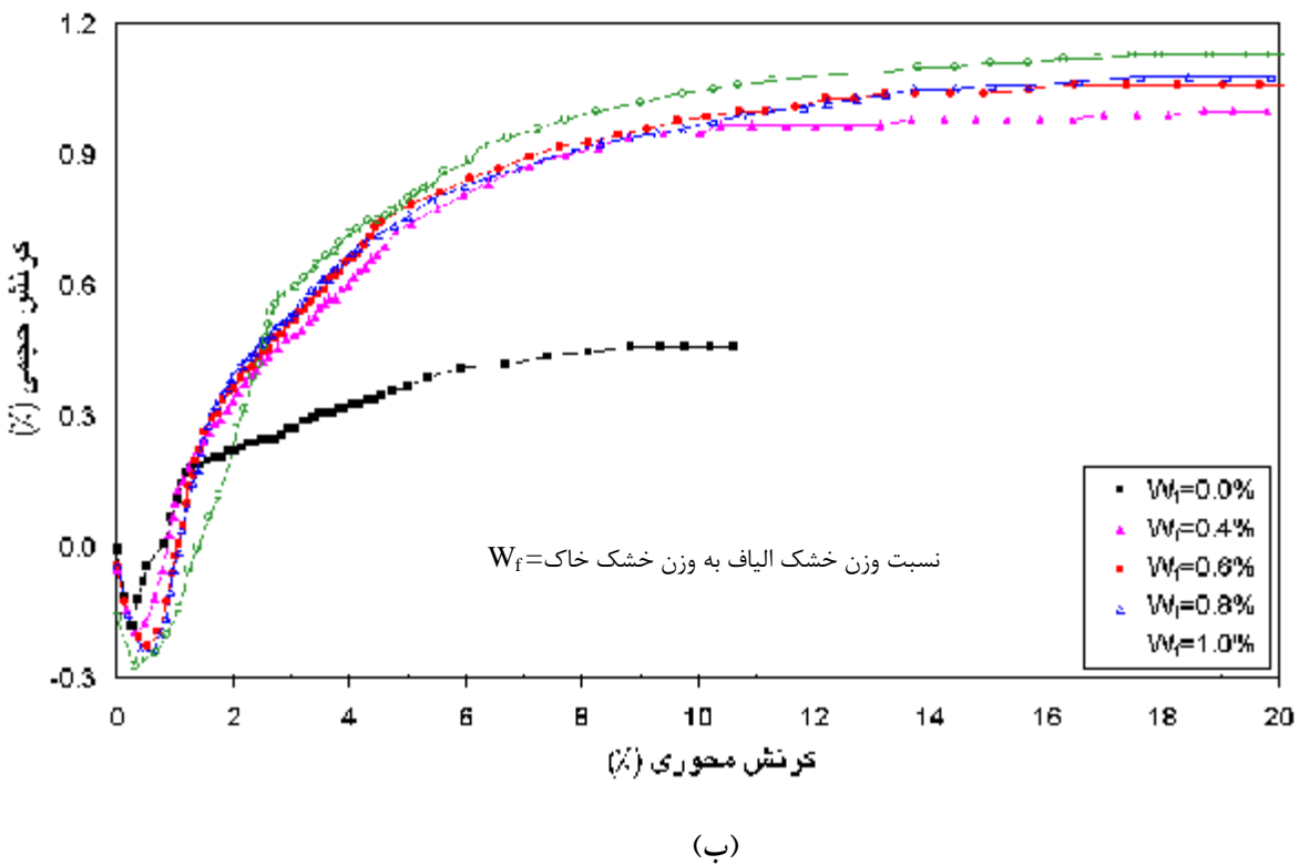
شکل ۶- تغییرات تنش انحرافی (شکل الف) و کرنش حجمی (شکل ب) در آزمایش سه محوری CD ( s'_c = 100 \text{ kPa} ) برای درصدهای وزنی مختلف عناصر تسلیح ( W_f ) و نسبت اضلاع عناصر A_R = 9
