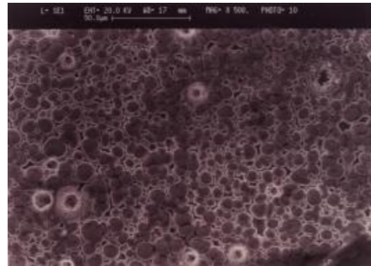
شکل ۲- تصویر SEM از سطح پوشش حاصل از روش مستقیم با ترکیب آلیاژی Zn=0.52/8 و Ni=0.47/2 و شرایط آبکاری I=11 \text{ A/dm}^2 ; T=60^\circ \text{C} ; pH=00 ۲ نحوهٔ رشد پوشش و ایجاد حفره
