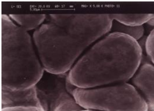
شکل ۲- تصویر SEM از سطح پوشش حاصل از روش مستقیم با ترکیب آلیاژی Zn=0.52/8 و Ni=0.47/2 و شرایط آبکاری I=11 \text{ A/dm}^2 ; T=60^\circ \text{C} ; pH=00 ۲ نحوهٔ رشد پوشش و ایجاد حفره
