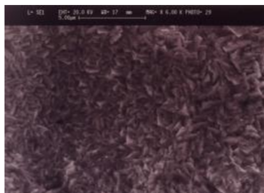
شکل ۳- تصویر SEM از سطح پوشش حاصل از روش منقطع با ترکیب آلیاژی Zn=0.81/7 و Ni=0.18/3 و شرایط آبکاری f=170 \text{ HZ} ; t_{on}=2/4 \text{ m sec} ; \text{On-Time}=0.40 ; I_{peak}=40 \text{ A/dm}^2
