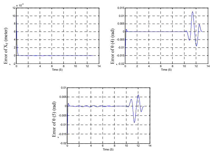
شکل ۱۴- خطای برخی از مختصات تعمیم یافته بر حسب زمان با اعمال الگوریتم کنترلی MBA با در نظر گرفتن اغتشاش محیطی
