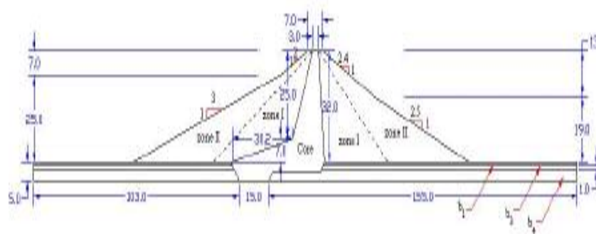
شکل ۲۴- مقطع عرضی سد "کارسینگتون"
