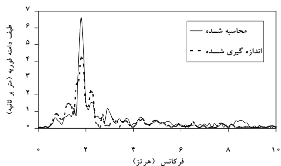
شکل ۲۱- طیف دامنه فوریه شتاب افقی در اثر زلزله "ماموت لیک" در تاج سد "لانگولی"
