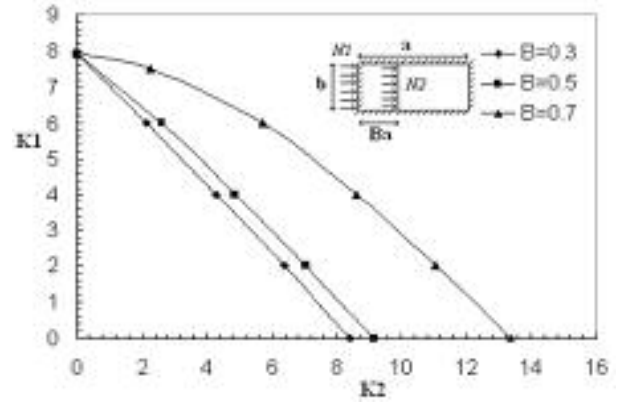
شکل ۹ - نمودار اندرکنش ضرایب کمانش k_1 و k_2 ( a=2b )
