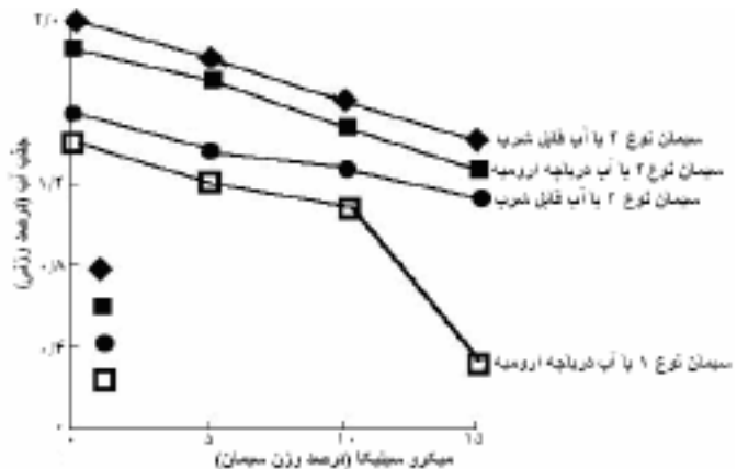
شکل ۱۵- تاثیرات نوع سیمان و مقدار میکروسلیس بر جذب آب مخلوطها در آبهای معمولی و دریاچه ارومیه
