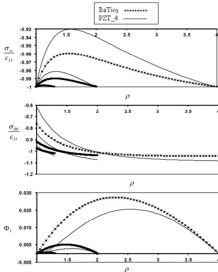
شکل ۶- حالت پنجم بارگذاری برای نسبت‌های شعاع \eta = 1, 3, 2, 4
