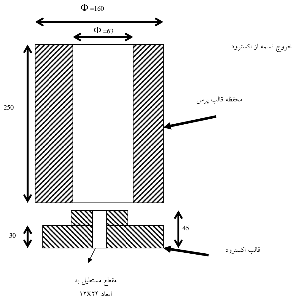
شکل ۳- نقشه مکانیکی مخزنه قالب پرس و قالب اکستروژن برای پرس پودر و اکستروژن گرم پیش ماده
