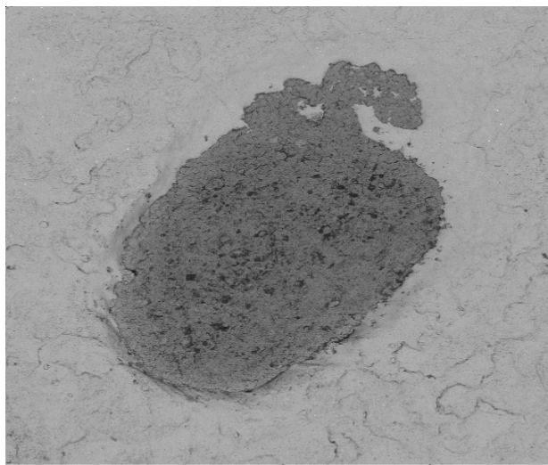
شکل ۳- نمونه نورد پوسته‌ای شده دارای عیب فاقد پوشش.
