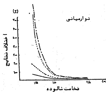
شکل ۹- اثر افزایش ضخامت شالوده بر M_y
