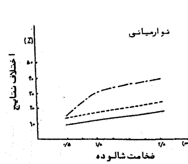
شکل ۸- اثر افزایش ضخامت شالوده بر M_x
