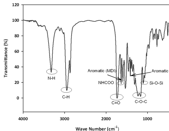
شکل ۲- طیف FTIR فیلم پلیمری POSS/PCU
