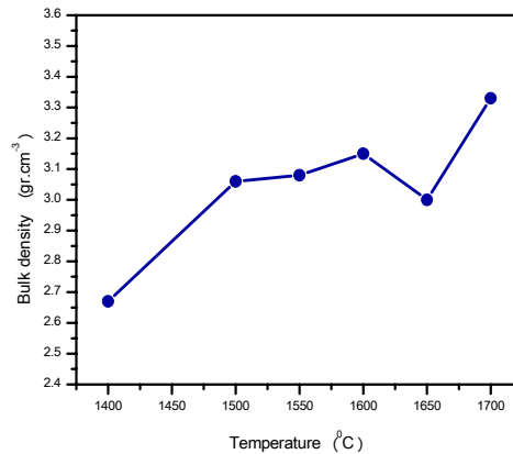
شکل ۷- تغییرات دانسیته کلی نمونه در دماهای مختلف زیتتر
