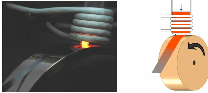
شکل ۱- طرح شمایی و تصویر فرایند ریخته رسی [۴].
