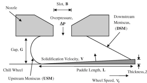
شکل ۱- طرح شمایی و تصویر فرایند ریخته رسی [۴].
