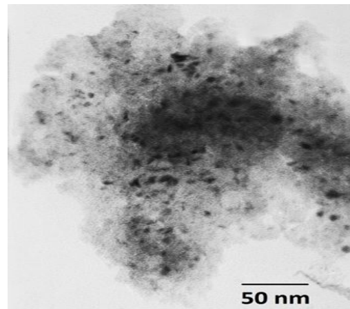
شکل ۶- تصویر میکروسکوپ الکترونی عبوری نمونه ۲۰ ساعت آسیاب شده
