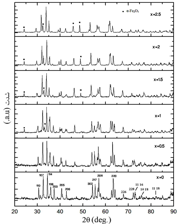
شکل ۴- الگوهای پراش پرتو ایکس نانو ذرات فریت استرانسیم با ترکیب \text{SrFe}_{12-2x}(\text{MgCo})_{0.5x}\text{Ti}_x\text{O}_{19} به ازای مقادیر مختلفی از x ، ساخته شده در دمای 900^\circ\text{C} درجه سانتی‌گراد به مدت ۱ ساعت
