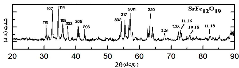
شکل ۳- الگوی پراش پرتو ایکس نمونه فریت استرانسیم در دمای 870^\circ درجه سانتی گراد به مدت ۱ ساعت
