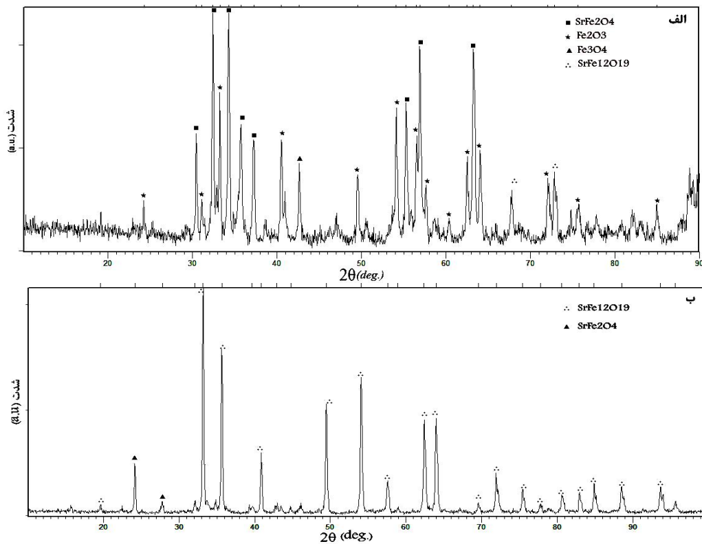
شکل ۲- الگوهای پراش پرتو ایکس فریت استرانسیم ساخته شده در دمای الف) 700^\circ و ب) 800^\circ درجه سانتی گراد به مدت ۱ ساعت
