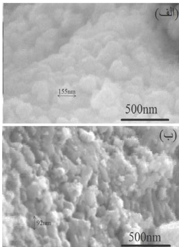
شکل ۳- تصاویر میکروسکوپ الکترونی روبشی گسیل میدانی (FE-SEM): الف) نمونه Ag-TiO 2 و ب) نمونه ZnO-TiO 2
