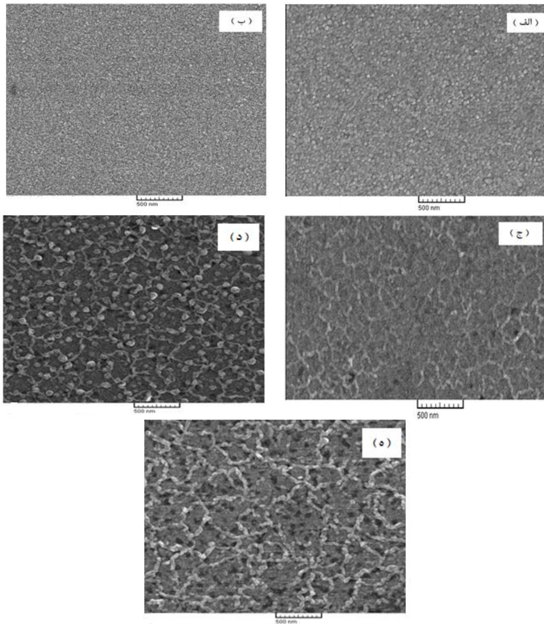
شکل ۳- تصاویر میکروسکوپی لایه‌های نازک نئودمیوم-آهن-بور در دمای آنیل مختلف: الف) ۴۵۰، ب) ۵۰۰، ج) ۵۵۰، د) ۶۰۰ و ه) ۶۵۰ درجه‌سانتی‌گراد
