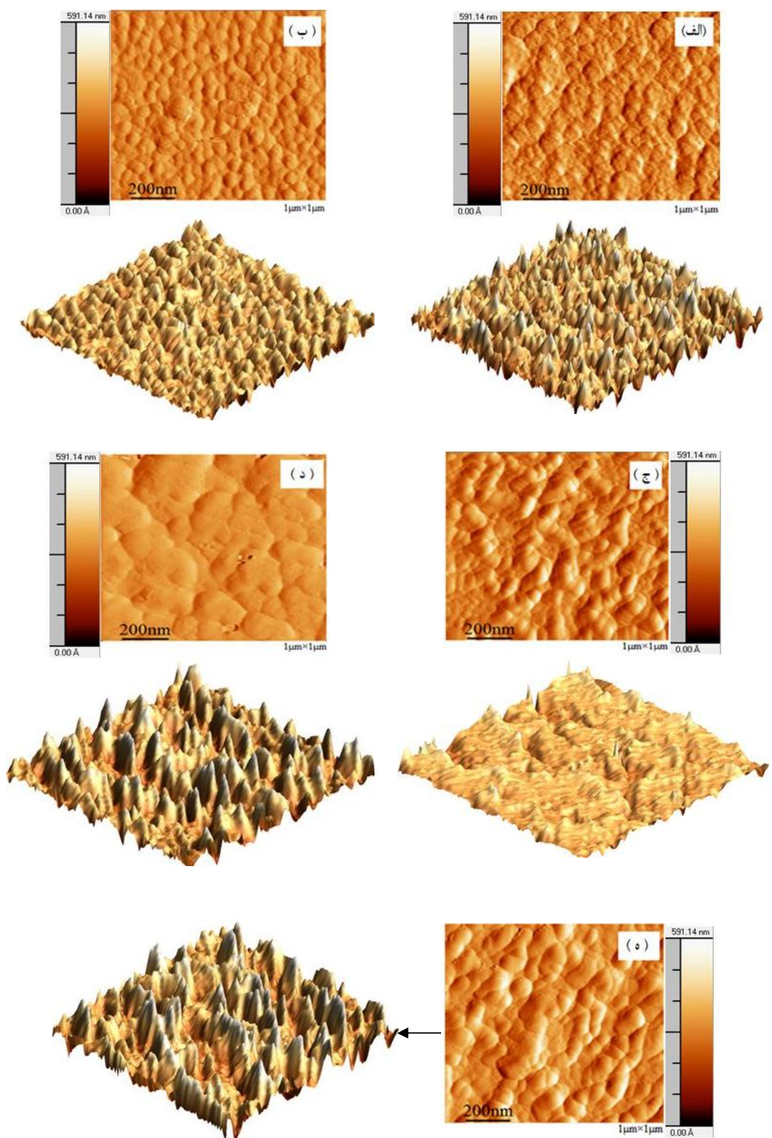
شکل ۴- تصاویر میکروسکوپی روبشی لایه‌های نازک نئودیمیوم آهن بور در دمای آنیل مختلف: الف) (۴۵۰، ب) (۵۰۰، ج) (۵۵۰، د) (۶۰۰ و ه) (۶۵۰ درجه سانتی‌گراد
