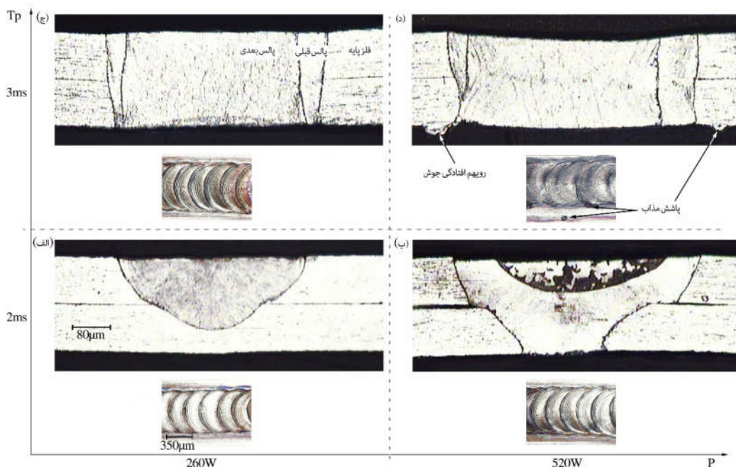
شکل ۵- تصاویر میکروسکوپی نوری از مقطع و سطح جوش در f=1\text{Vs}^{-1} (الف: P=260\text{W} و T_p=2\text{ms} و ب: P=520\text{W} و T_p=2\text{ms} ، ج: P=260\text{W} و T_p=3\text{ms} و د: P=520\text{W} و T_p=3\text{ms} )
