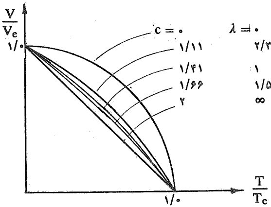
شکل ۳ - منحنی تسلیم اولیه پایه صلب لغزشی بر حسب مقادیر مختلف نسبت ابعاد
