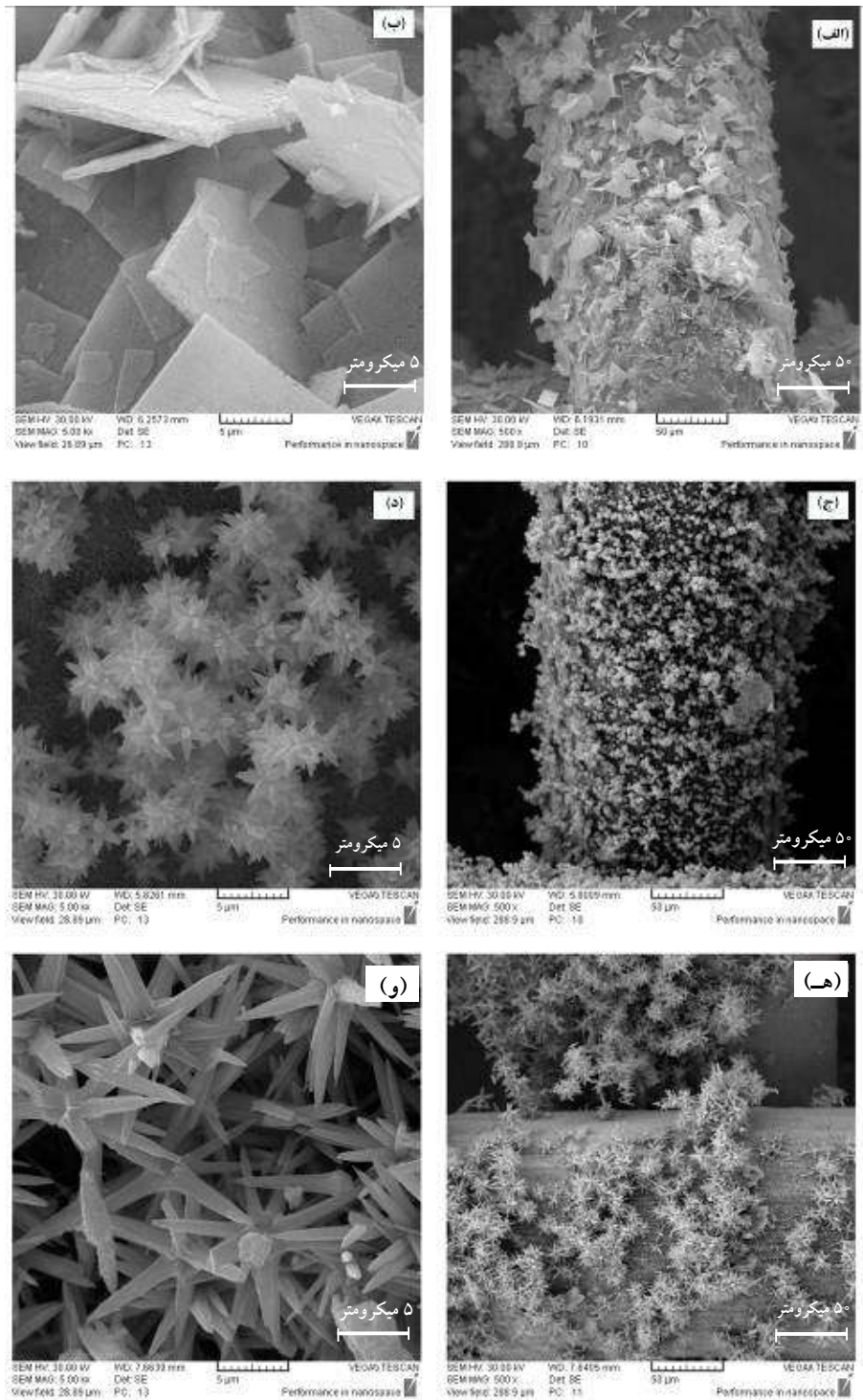
شکل ۳- تصاویر میکروسکوپی الکترونی روبشی از سطح ZnO تهیه شده با استفاده از آمونیاک به عنوان عامل بازی در مرحله سنتز: الف) و ب) بدون حضور پلی اتیلن گلیکول، ج) و د) غلظت ۰/۲۵ میلی مولار پلی اتیلن گلیکول، ه) و و) غلظت ۰/۰۵ میلی مولار پلی اتیلن گلیکول
