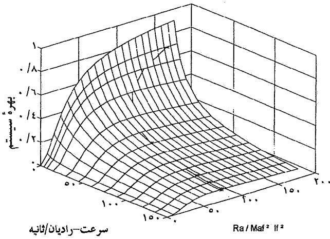
شکل ۲۲- بهره سیستم در موتور تحریک جداگانه حداکثر آن در سرعت ثابت: -۰-
