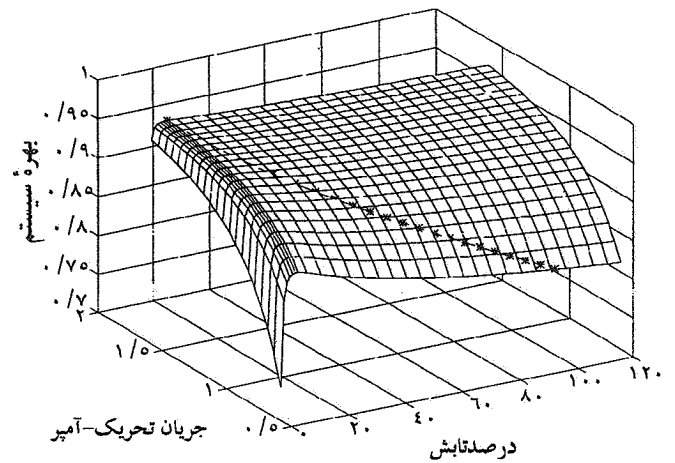
شکل ۲۱- بهره سیستم در موتور تحریک جداگانه همراه با مرز مبدل‌های افزایشنده و کاهشنده: -۰-
