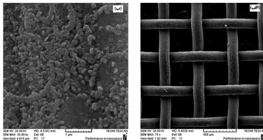
شکل ۱- تصاویر میکروسکوپی الکترونی روبشی از سطح توری استیل: الف) توری خام و ب) بعد از ایجاد بذر لایه
