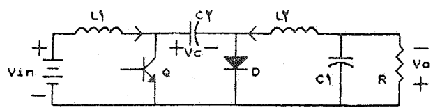
شکل ۷- مبدل چوک
