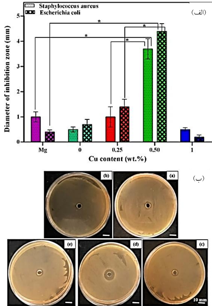
شکل ۶- خاصیت آنتی‌باکتریال منیزیم و آلایزهای Mg-1Al-Cu حاوی مقادیر مختلف مس (صفر، ۰/۲۵، ۰/۵ و ۱ درصد وزنی)، (الف) نمودار تغییرات قطر هاله عدم رشد و (ب) هاله رشد تشکیل شده در اطراف نمونه‌ها (*: اختلاف معنادار بین گروه‌ها (P < ۰/۰۵))
