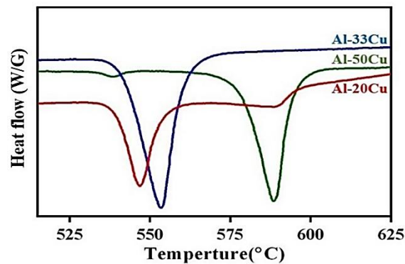
شکل ۲- نمودار آنالیز حرارتی افتراقی پودرهای آلومینیوم و مس آسیا شده به مدت ۲۰ ساعت
