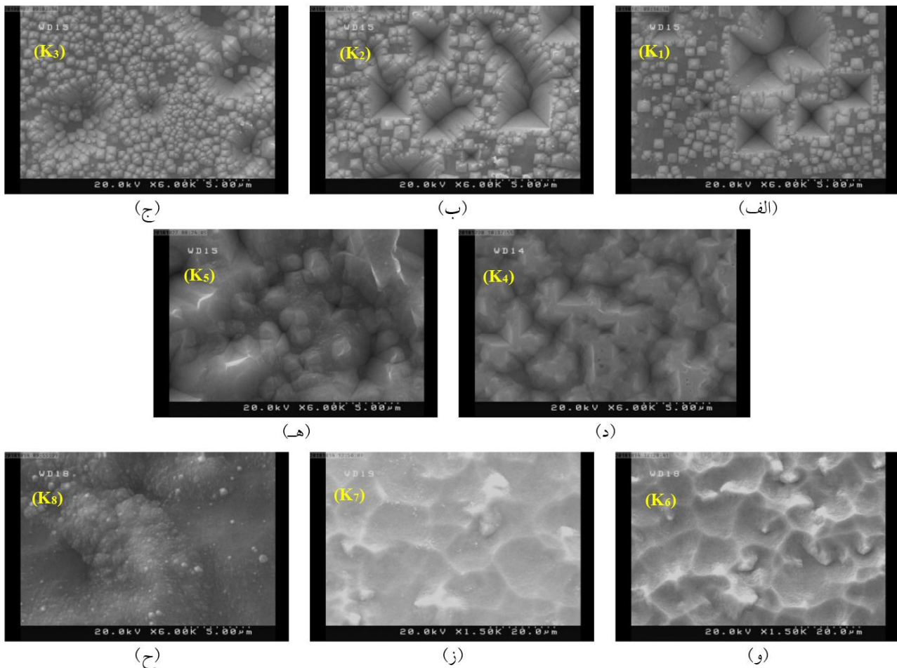
شکل ۷- ساختارهای شکل گرفته بر بستر سیلیکونی در محلول نیترات مس 0.005\% مولار و هیدروفلوئوریک اسید 4/6 مولار در دمای 50^\circ درجه سانتی‌گراد (به همراه پس‌زدایش) به مدت زمان‌های: الف) 10 ثانیه، ب) 20 ثانیه، ج) 30 ثانیه، د) 1 دقیقه، ه) 2 دقیقه، و) 3 دقیقه، ز) 4 دقیقه و ح) 5 دقیقه
