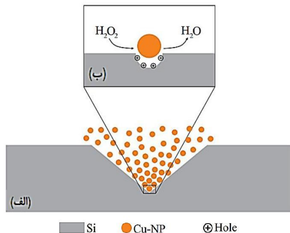
شکل ۱- الف) رسوب نانوذرات مس روی بستر سیلیکونی و شکل‌گیری ساختارهای نانوهرم وارونه و ب) فرایند کاهش هیدروژن پراکساید و شکل‌گیری گودال روی بستر سیلیکونی
