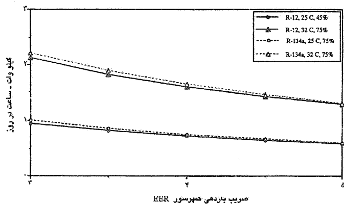
شکل ۵- تاثیر استفاده از کمپرسورهای با بازده بالاتر روی مصرف برق یخچال نمونه
