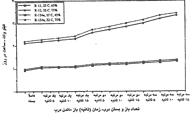
شکل ۹- تاثیر تعداد دفعات باز و بسته کردن درب روی مصرف انرژی یخچال نمونه
