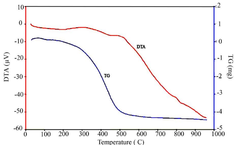
شکل ۲- منحنی گرماوزن‌سنجی /حرارتی تفاضلی مربوط به ژل خشک شده نمونه S75
