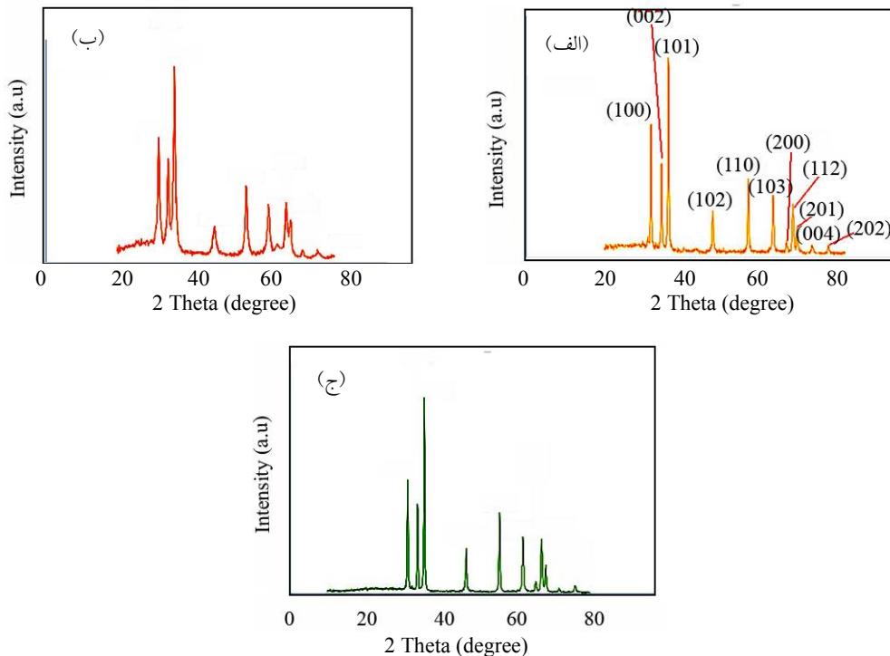
شکل ۴- الگوی پراش پرتو ایکس نمونه S75 سنتز شده در دمای کلسینه: (الف) ۵۰۰ درجه سانتی گراد، (ب) ۶۰۰ درجه سانتی گراد و (ج) ۷۰۰ درجه سانتی گراد
