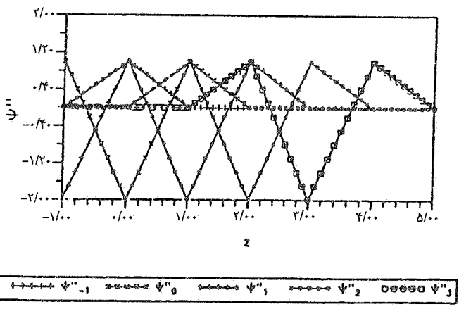
شکل ۴- مشتق مرتبه دوم تابع اسپلاین
