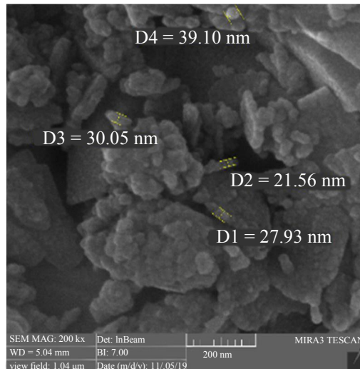
شکل ۹- تصویر میکروسکوپی الکترونی روبشی گسیل میدانی پودر سنتز شده در محیط گاز آرگون
