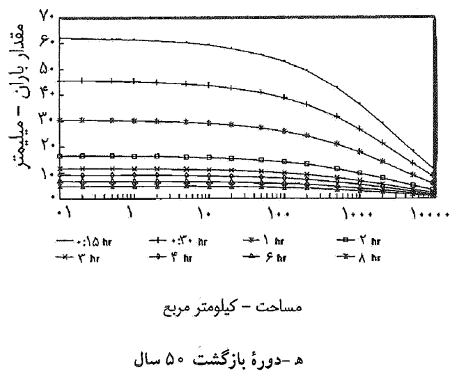
شکل ۷- دسته منحنیهای IDFA شهر مشهد
