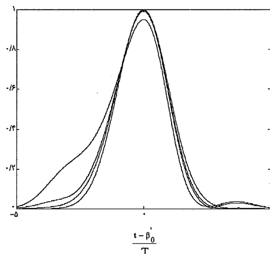
شکل ۵- پیش‌بینی پاره‌ای از اوج‌جهای امکانپذیر توسط پاشندگی ماده در یک فیبر نوری به طول ۱۰ کیلومتر در حوالی طول موج پاشندگی صفر (براساس الگوریتم پیشنهادی)
