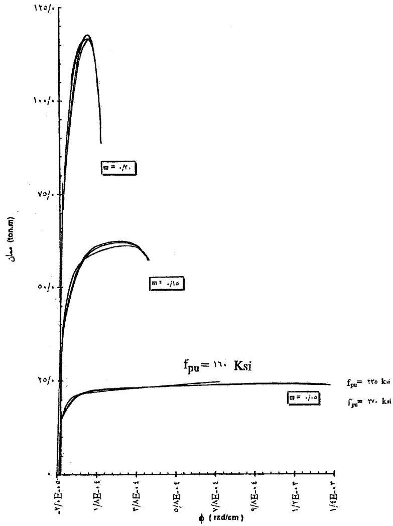
شکل ۱۷- اثر مقاومت نهایی فولاد پیش تنیده روی منحنی میان - انحنا برای فولادگذاری مختلف
