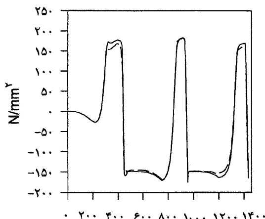
الف - توزیع تنش طولی
