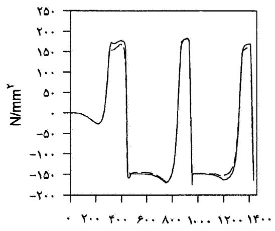
ب - توزیع کرنش طولی مسافت طی شده توسط نوار [ mm ]
