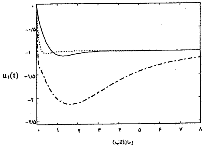
شکل ۷- سیگنال کنترل u_1(t) به ازای برخی از مقادیر نامعینها
