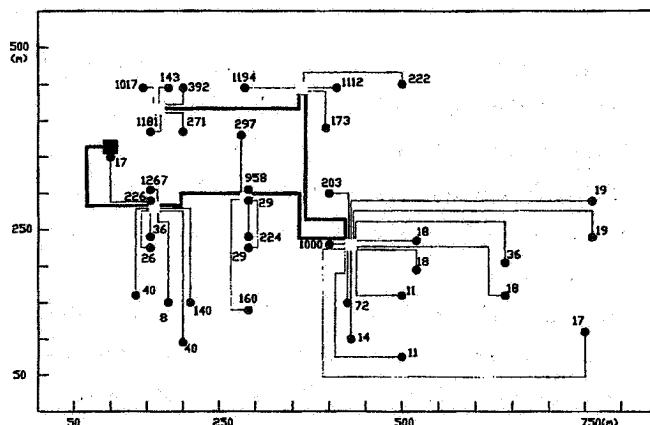
شکل ۷- طرح بهینه سیستم توزیع یک کارخانه شیمیایی. طرح بهینه ۱۲٪ از طرح نظری کم هزینه تر است. طرح نظری شامل ۱۱ پست توزیع بوده است.
