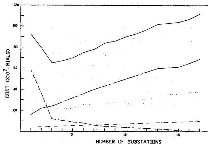
شکل ۹- منحنی هزینه‌های مختلف بر حسب تعداد پست فرعی در نمونه مورد مطالعه شماره (۲)
