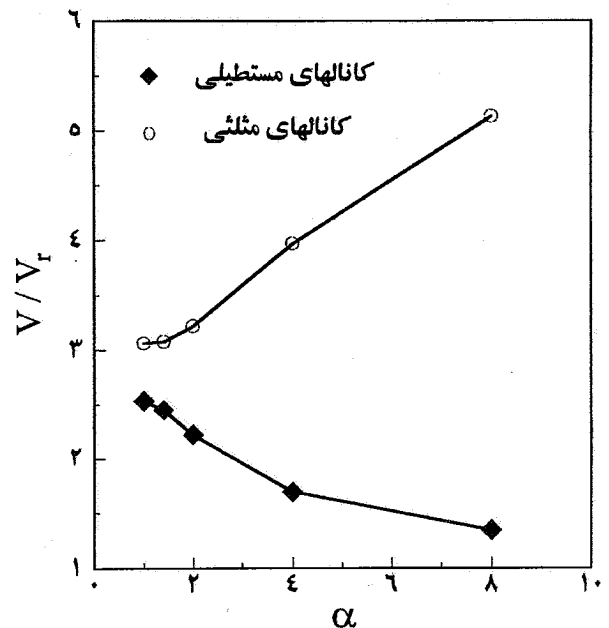
شکل 2- تغییرات نسبت حجم مبدل کانالهای مستطیلی و مثلثی به حجم مبدل سطح مینا بر حسب \alpha
