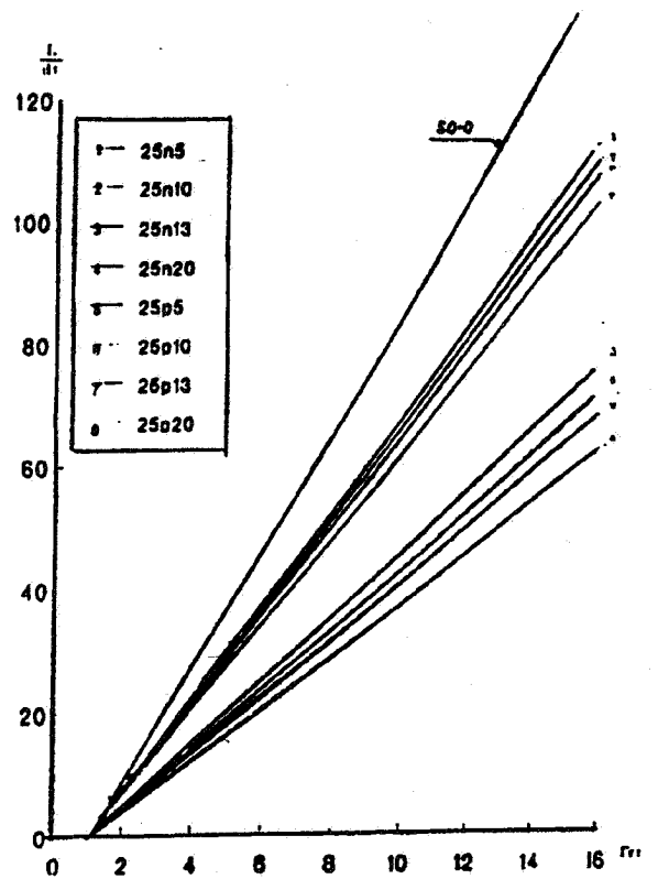
شکل ۹- مقایسه L/d_1 نسبت به Fr_1 بین پله‌های مثبت و منفی در شیبه‌های انتخابی
