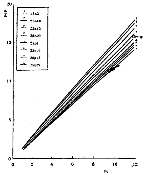
شکل ۸- مقایسه d_2/d_1 نسبت به Fr_1 بین پله‌های مثبت و منفی در شیبه‌های انتخابی
