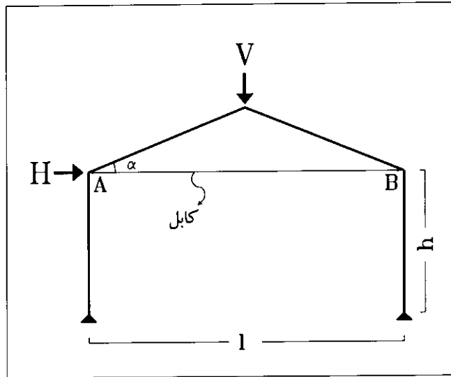
شکل ۱- سازه با کابل مهاری فقط کششی
