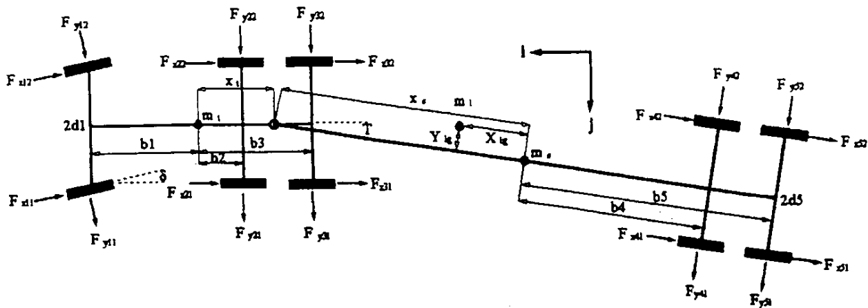
شکل ۳- مدل صفحه یاء و نیروهای مختلف خودرو
