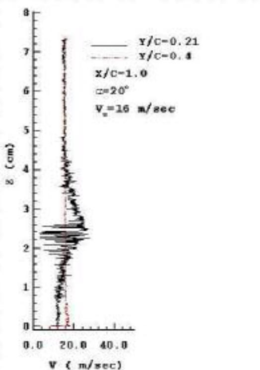
شکل ۹-ب- پروفیل سرعت لحظه‌ای در لبه فرار
