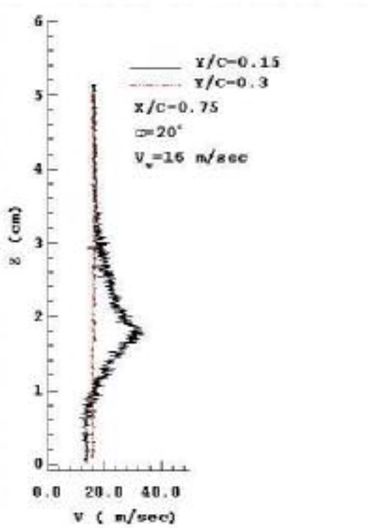
شکل ۹-الف- پروفیل سرعت لحظه‌ای در ۰/۷۵ وتر
